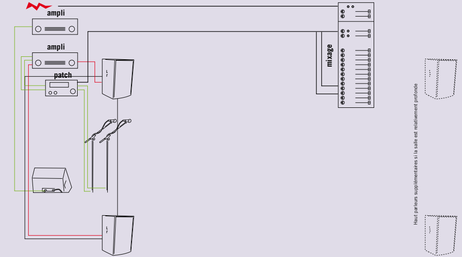
// SCHEMA D'INSTALLATION
